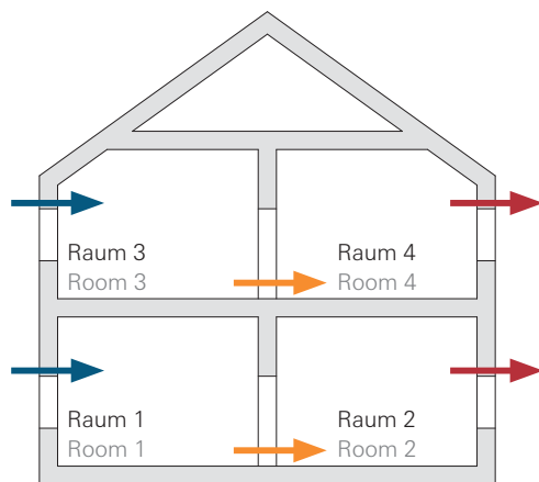
Beispiel 1: Querlüftung mit Außenluftdurchlässen Example 1: Cross ventilation with external air vents
