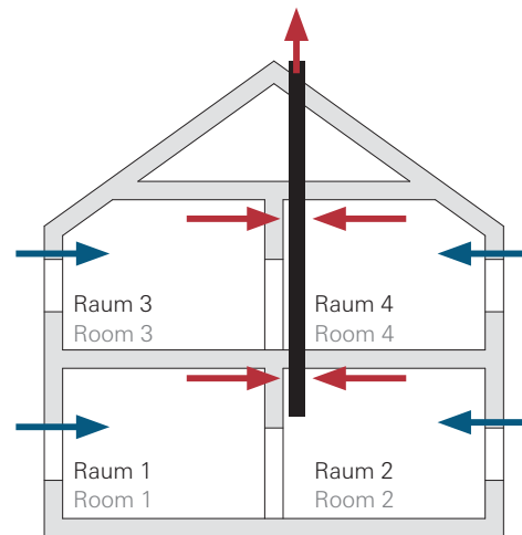
Beispiel 2: Abluftsystem mit Außenluftdurchlässen Example 2: Extraction system with external air vents
